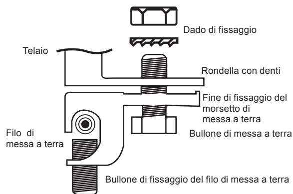
Figura 12 Metodo di messa a terra del bullone
