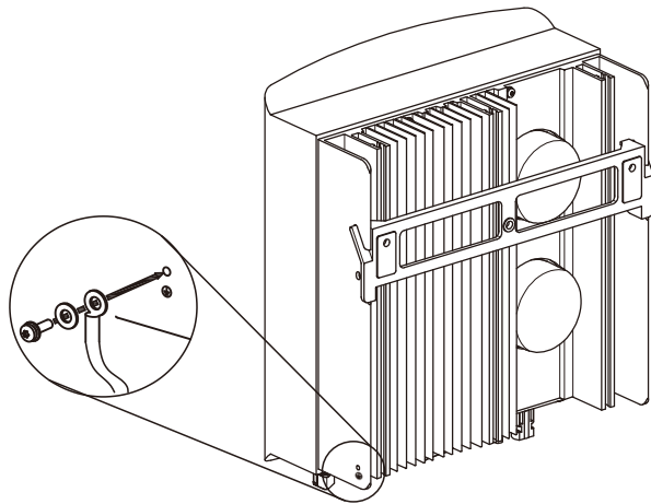
Figura 4.19 Collegare il conduttore di terra esterno
