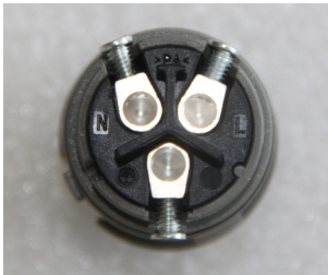
Figura 4.13 Connettore del terminale di rete CA all'interno
