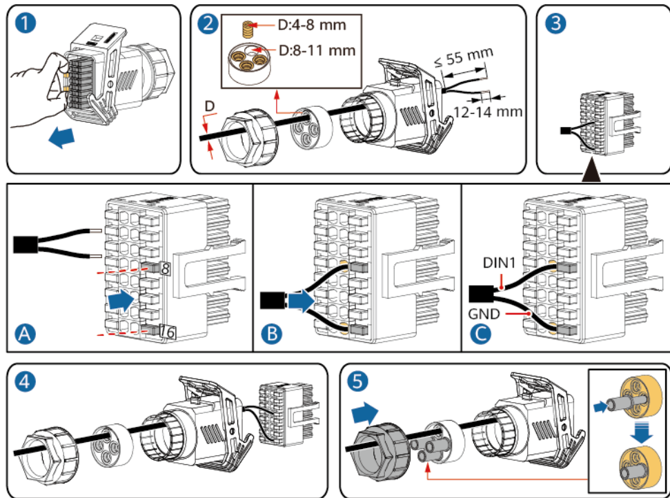
Figura 5-36 Installazione del cavo
