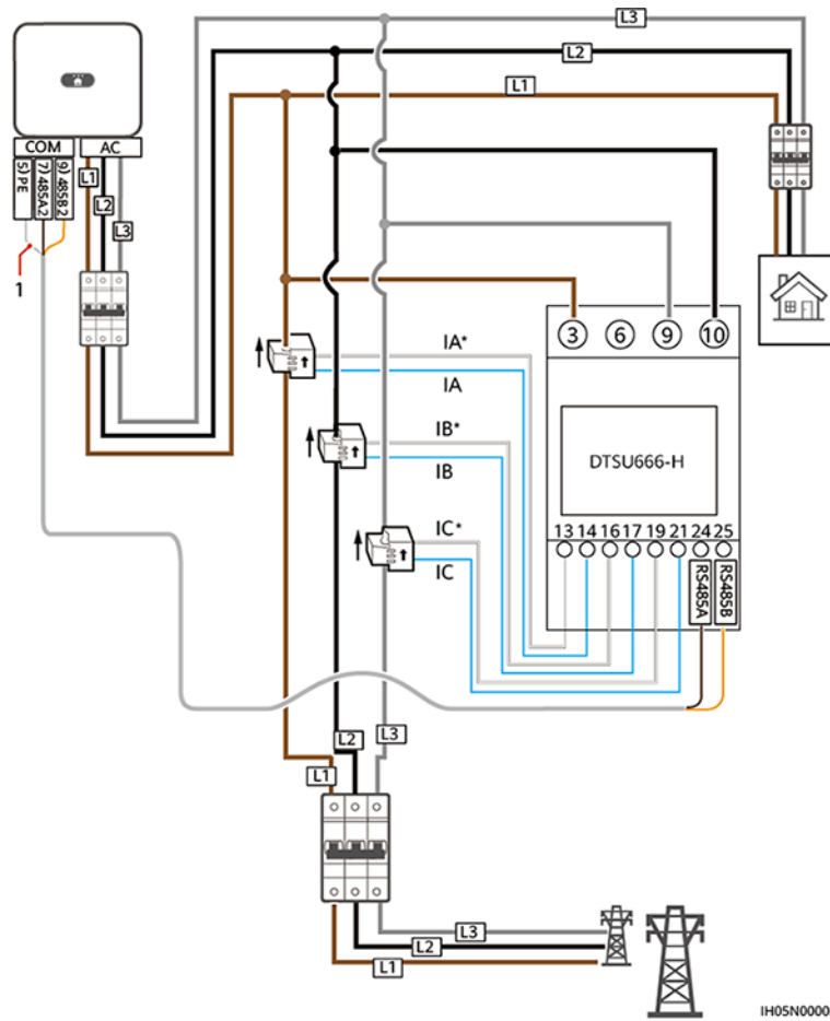
Figura 5-23 Connessione trifase, tre fili (rete di Smart Dongle)
