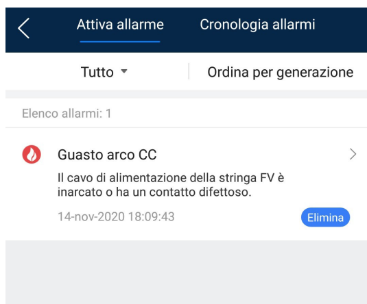
Figura 7-15 Gestione allarmi
