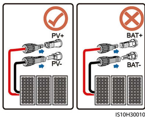
Figura 5-12 Terminali di cablaggio corretti
