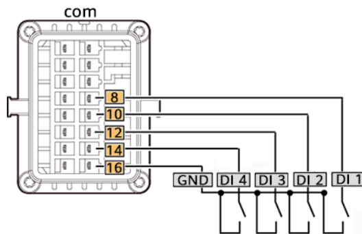
Figura 5-33 Collegamento dei cavi
