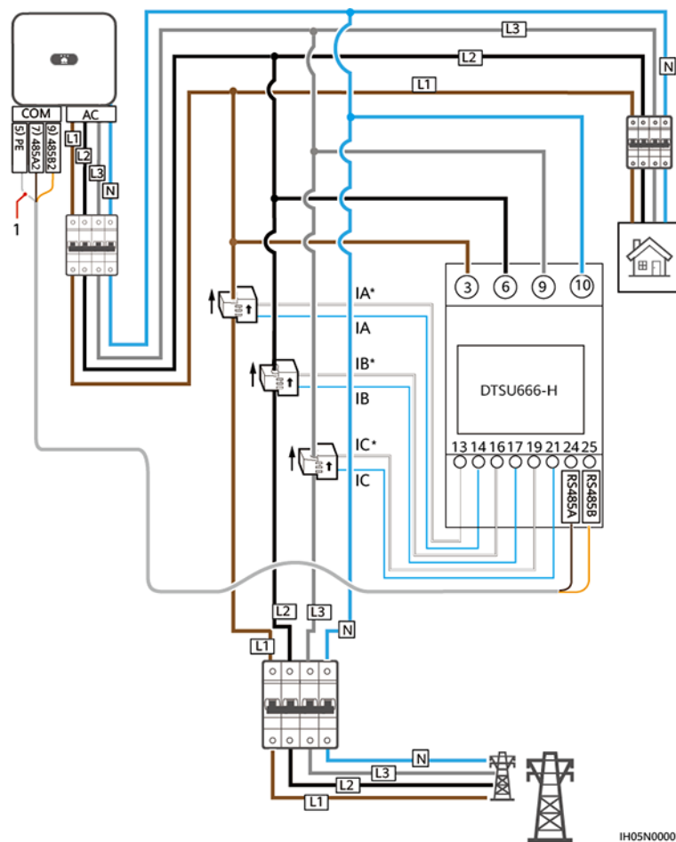
Figura 5-24 Connessione trifase, quattro fili (rete di Smart Dongle)
